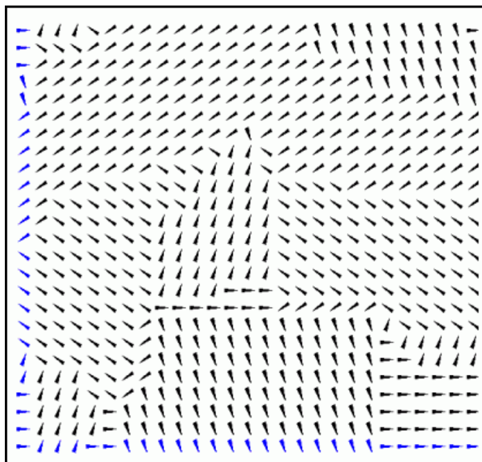
Weissovy domény v Pottsově modelu simulované Metropolisovou metodou. Při simulaci byly použity periodické okrajové podmínky (levá a pravá strana mají společné modré spiny, horní a dolní takéž).
